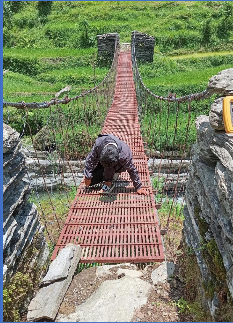
झोलुङ्गे पुल मर्मत
